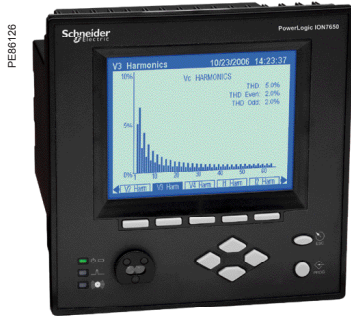
PowerLogic™ ION 7650.
