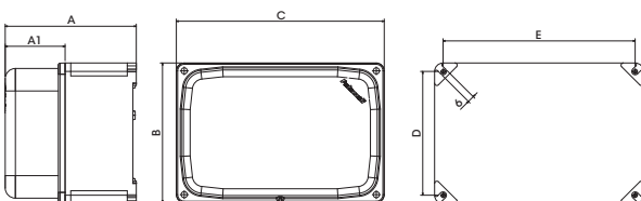
Boxes
