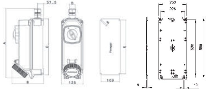
Sockets
